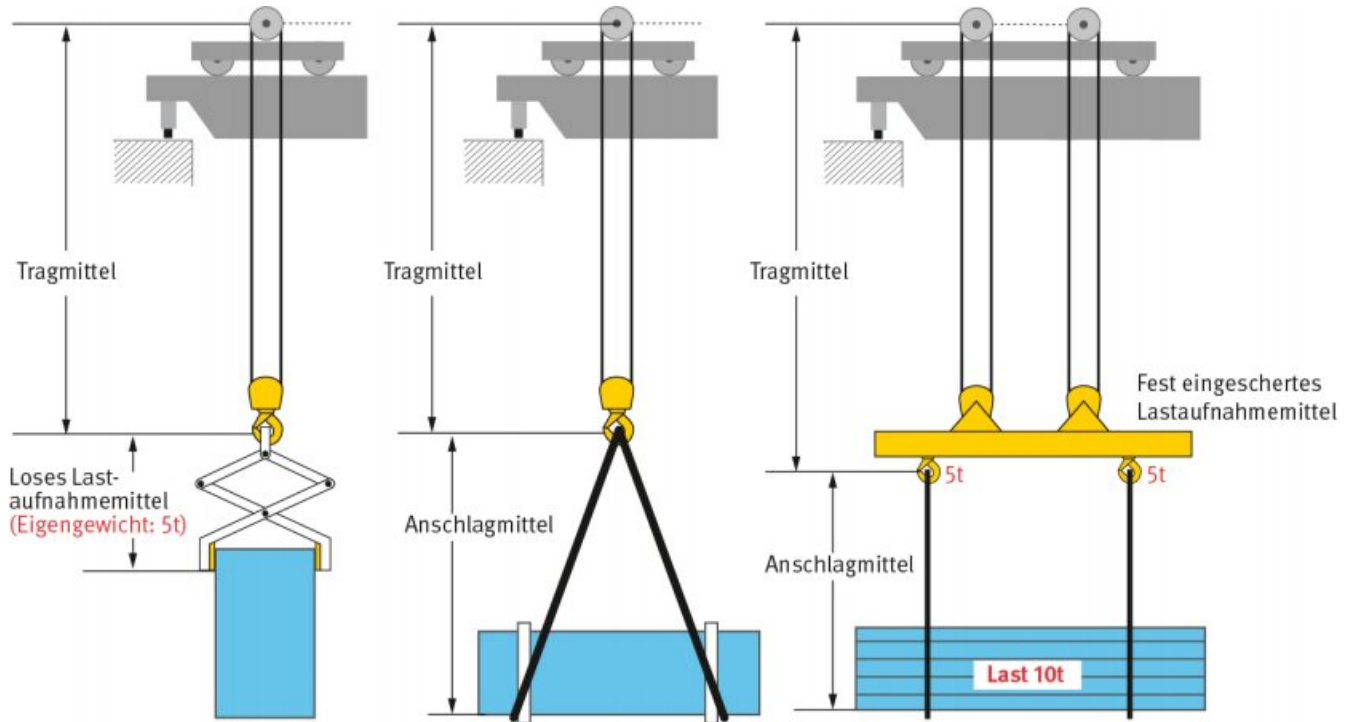
Abb.1 Darstellung von Lastaufnahmeeinrichtungen
